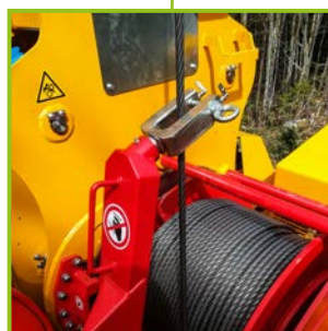
HYDRAULISCHE TS-EINLEITUNG
